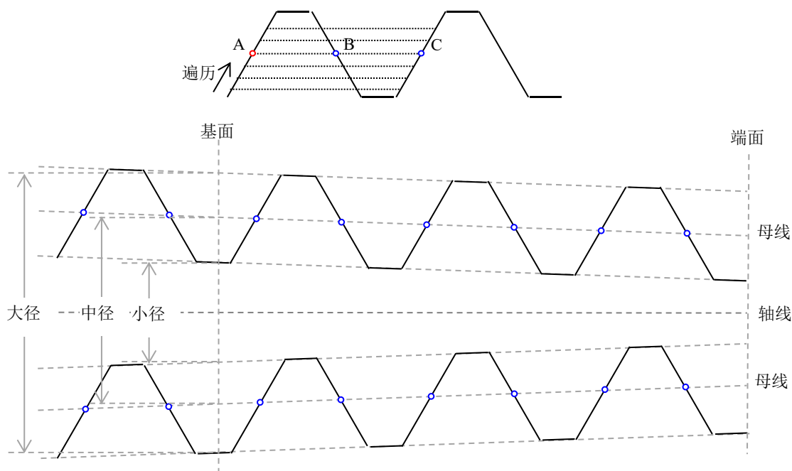
图 5 二维轮廓扫描法测量外螺纹基面中径
