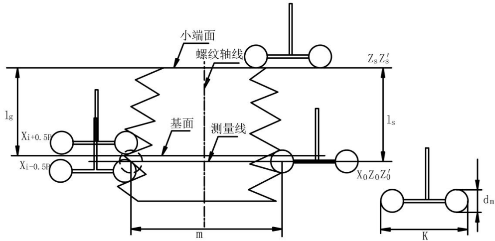
图 4.2 量球法测量外螺纹基面中径
