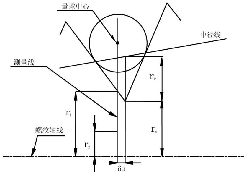
图 4.3 量球法测量外螺纹的轴向平面图
